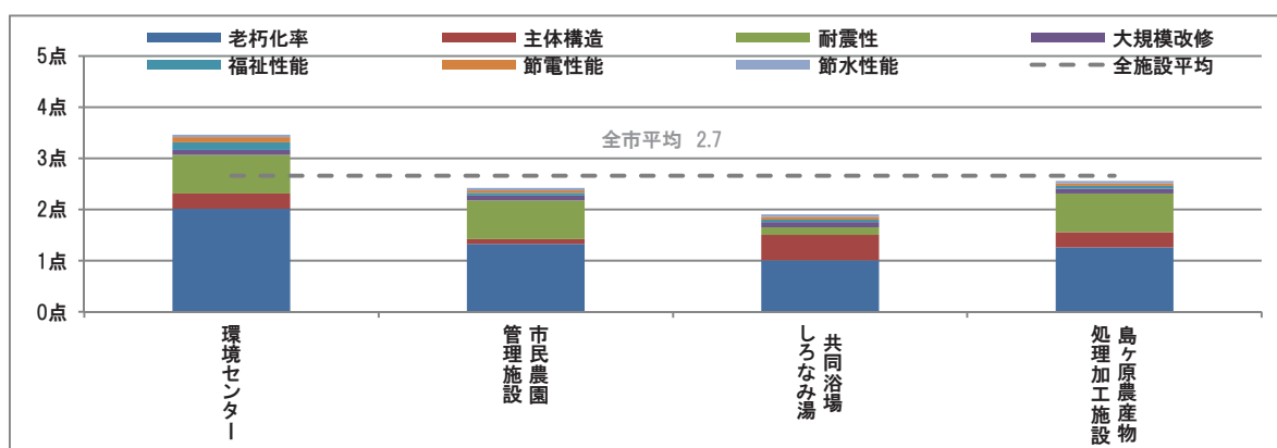
図 2-3-39 建物性能評価点の比較 (5点満点)
