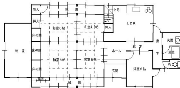
1 階 平面 図
