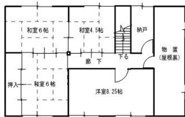
2階平面図
