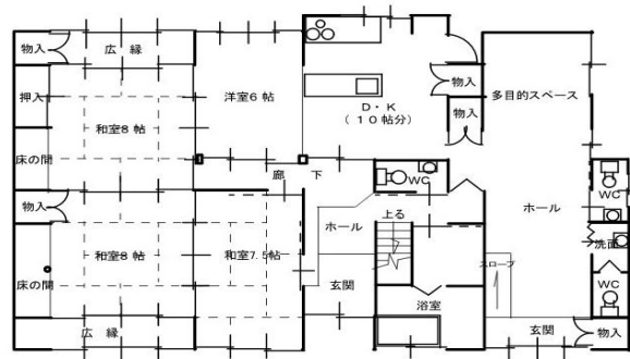
1階平面図 (全て賃貸可能)
