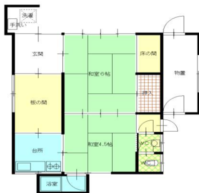
1階平面図
