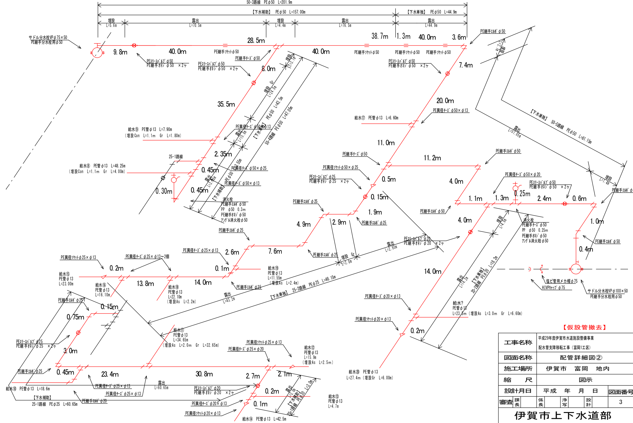
仮設配管詳細図 S=non
