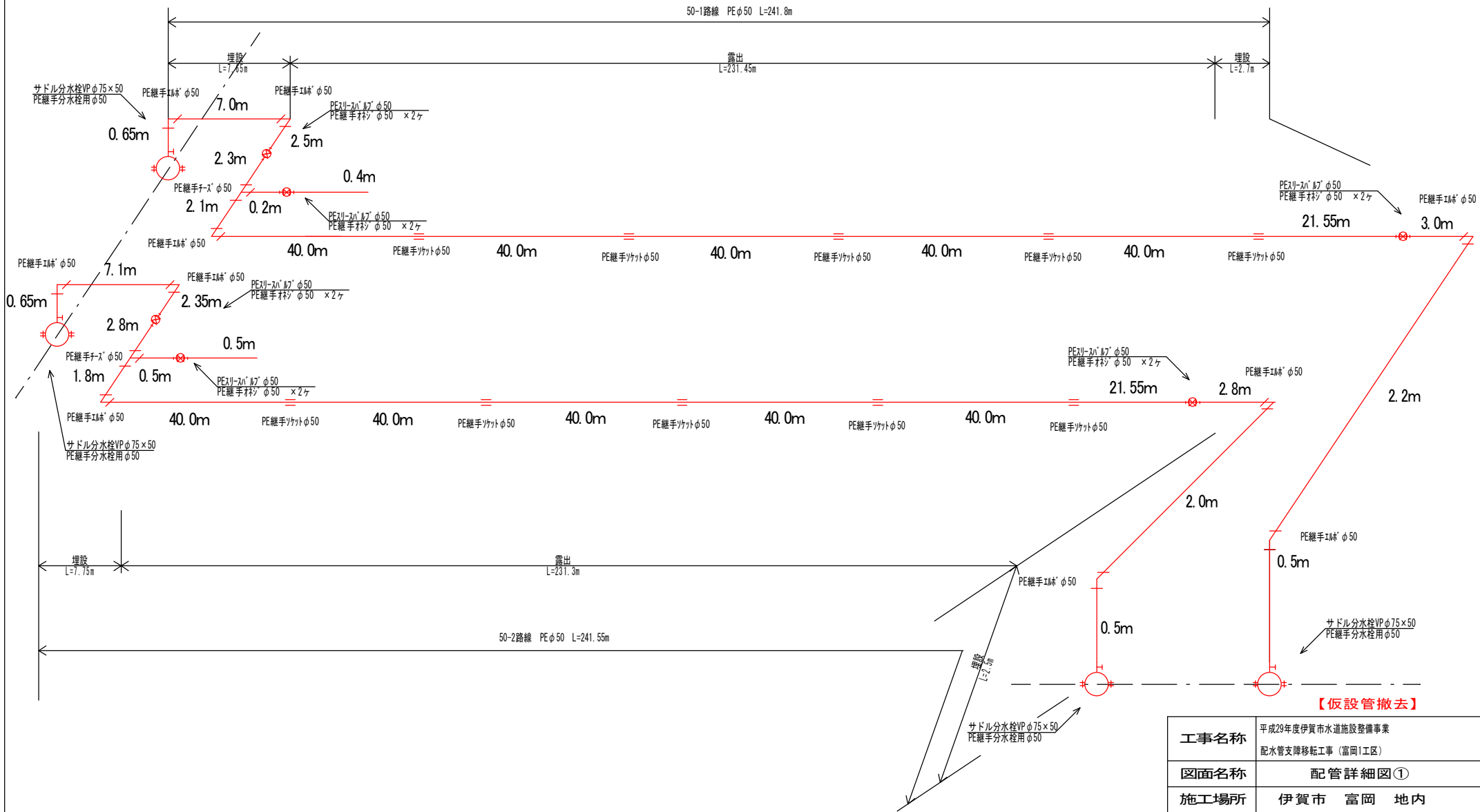
仮設配管詳細図 S=n o n
