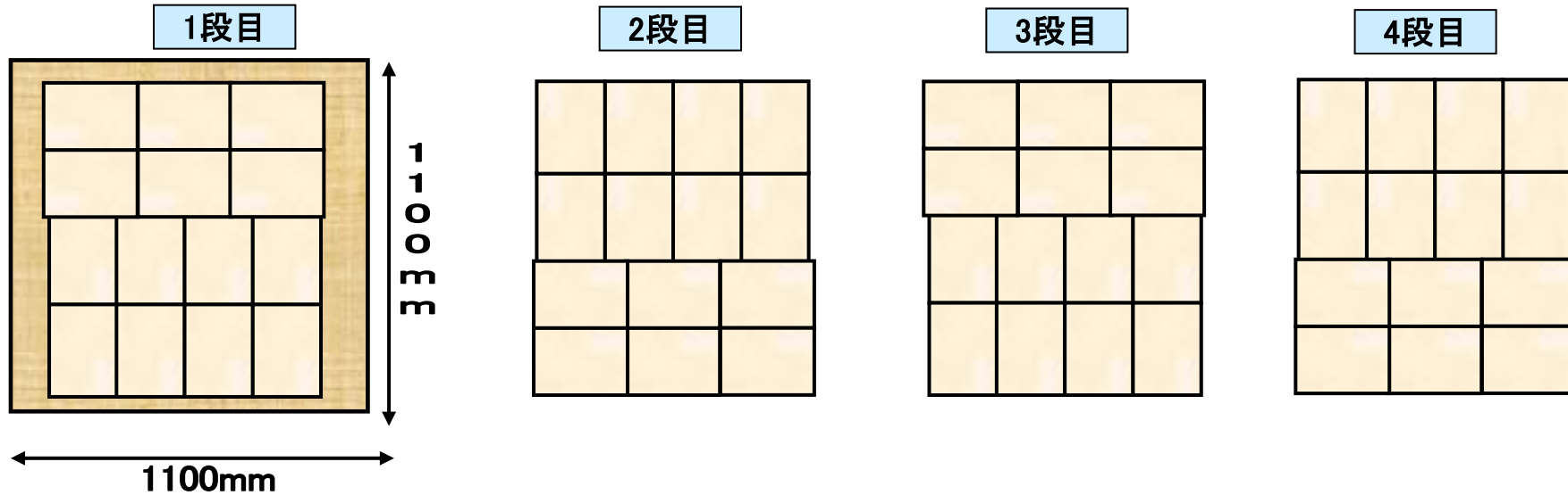
ダンボール箱仕様図
