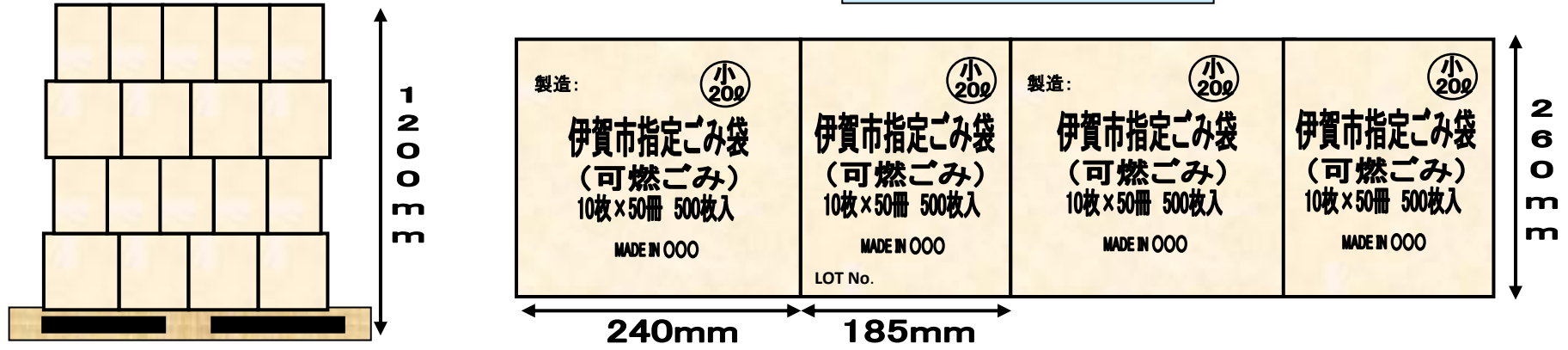
ダンボール箱仕様図
