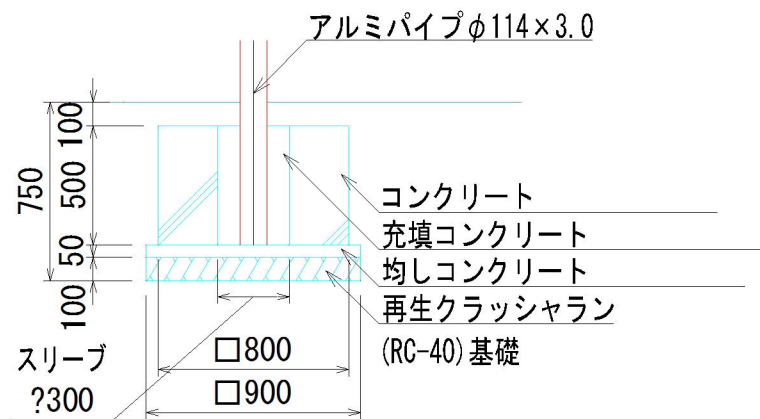
B' 基礎詳細図
