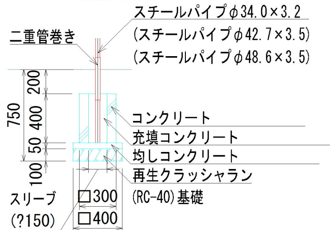
C' 基礎詳細図
