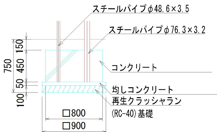
B基礎詳細図
