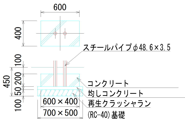
D基礎詳細図
