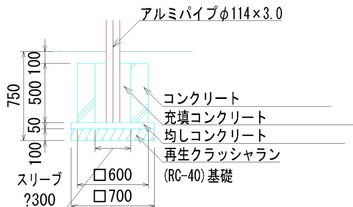
A' 基礎詳細図
