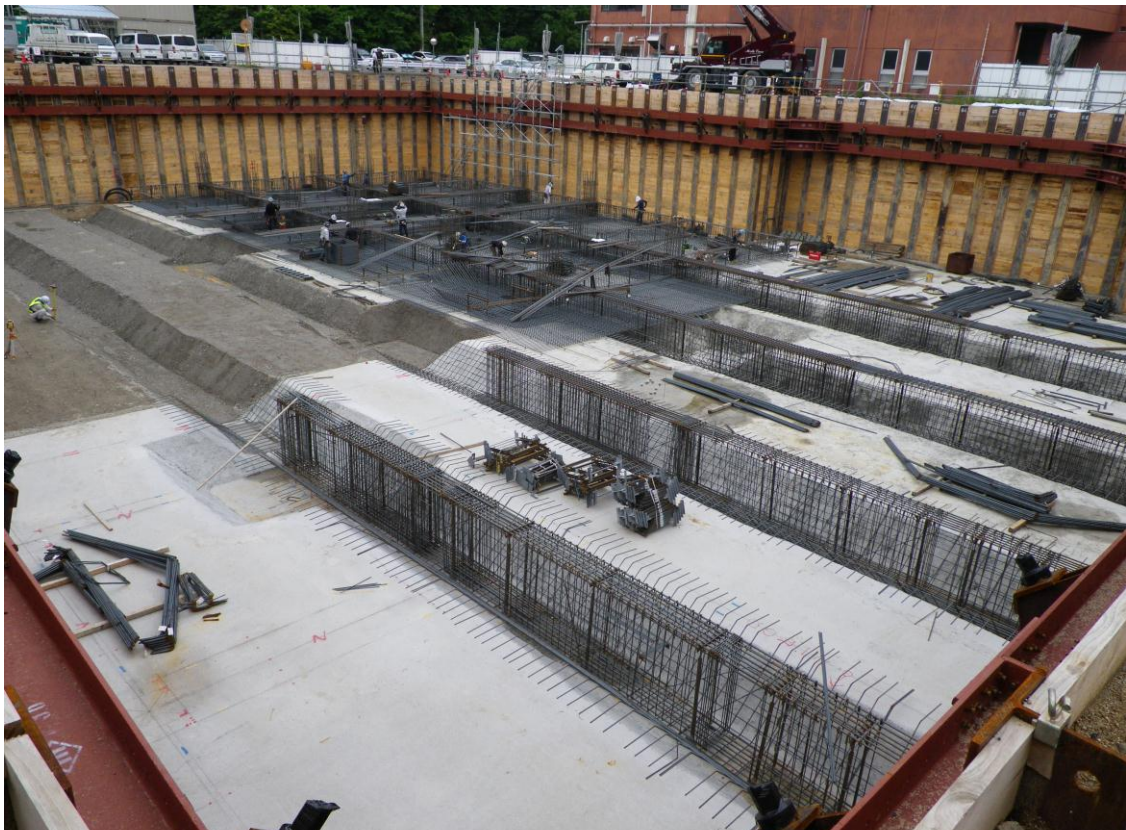
○基礎、配筋（北東端から）
