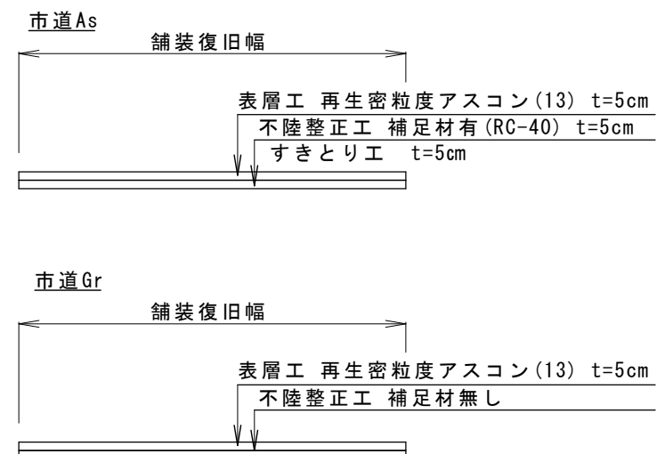
舗装本復旧標準図 S=1:20
