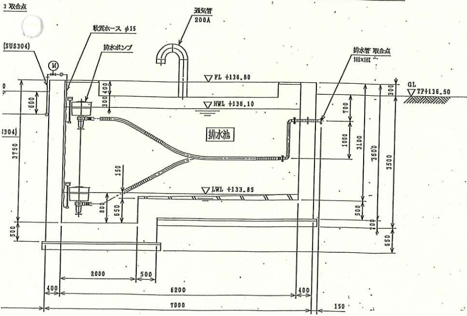
C-C断面図
