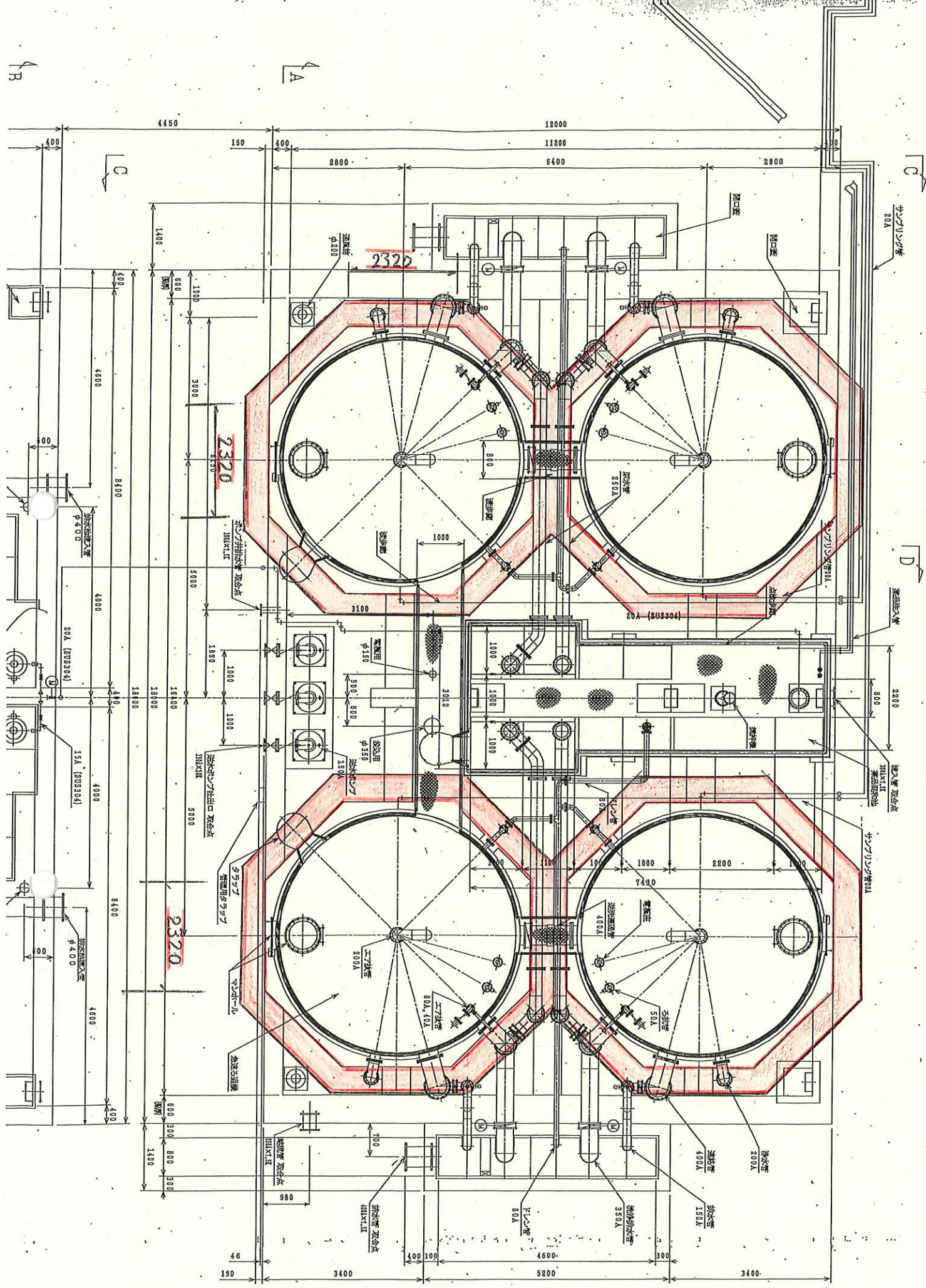
足場工平面図
