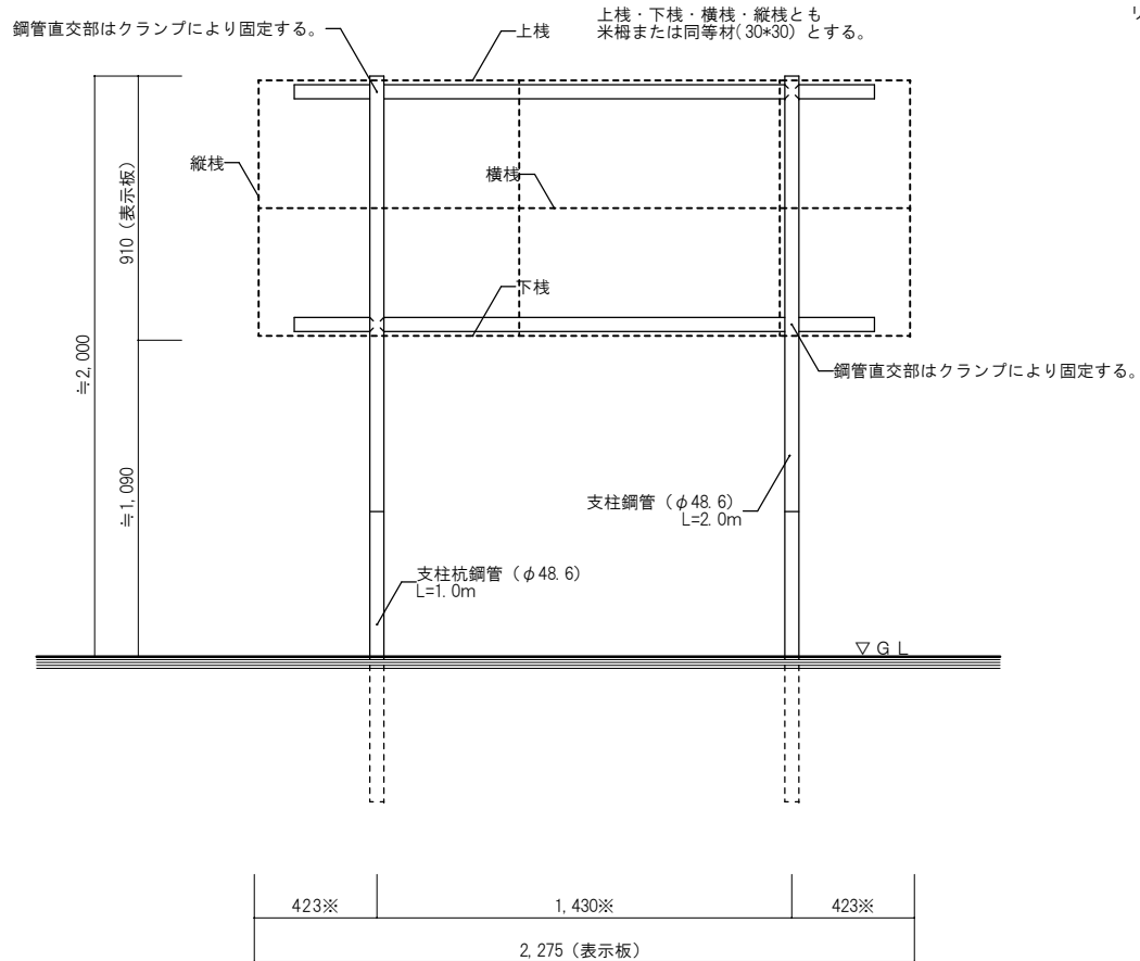
背面図 S = 1 : 20
