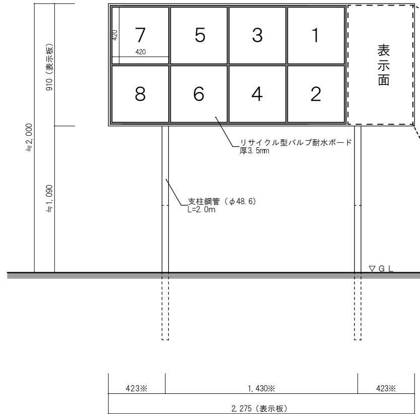
正面図 S = 1 : 20
