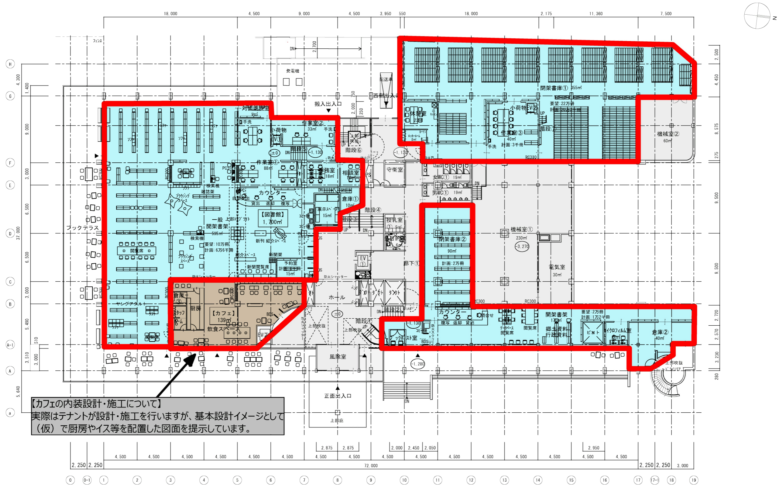
計画1階平面図 1/300
