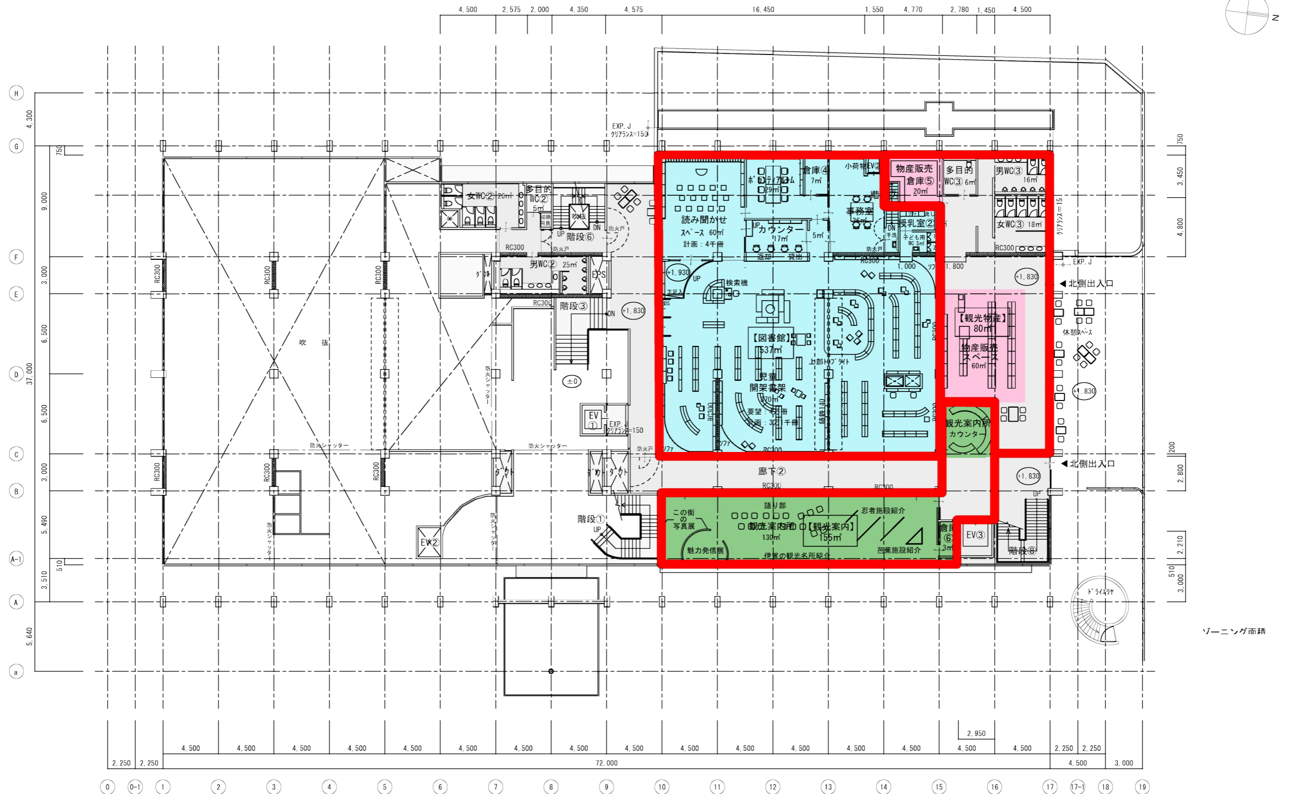
計画2階平面図 1/300
