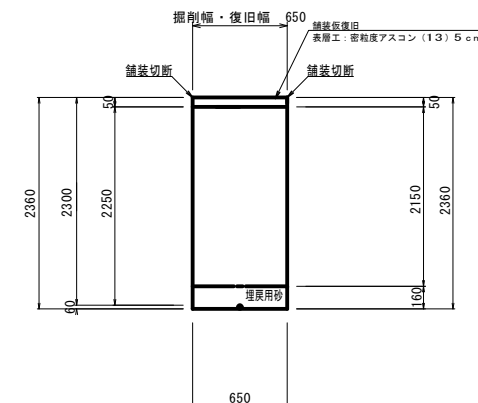
土工-5 (土被りH=2300) (PPφ50以下) 矢板有り
