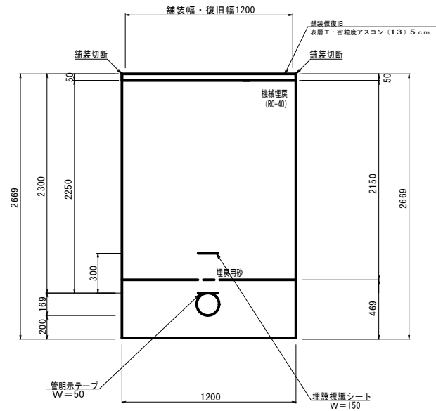
土工 -1 ( 不断水仕切弁 ) (土被りH=2300) (DCPφ150) 矢板有り
