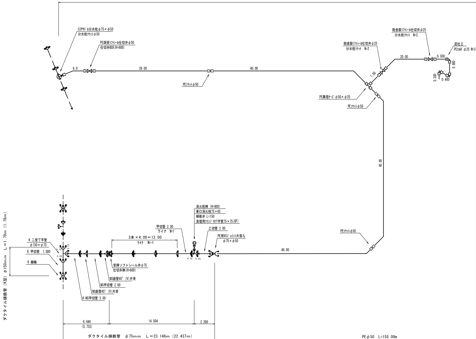
管割図
