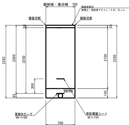
± 工 - 3 - 3 (土被りH=2300) (DCP φ 75) 矢板有り
