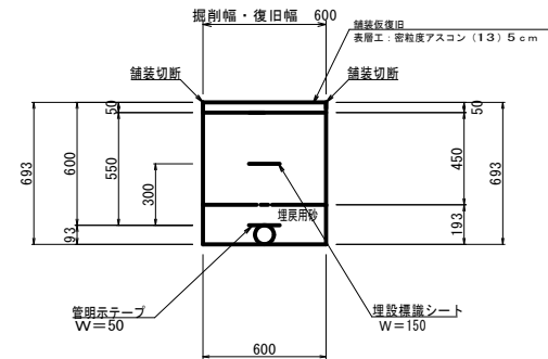
土工-3-1 (土被りH=600) (DCP φ75)
