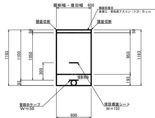
土 工 - 3 - 2 (土被りH=1100) (DCP φ 75)
