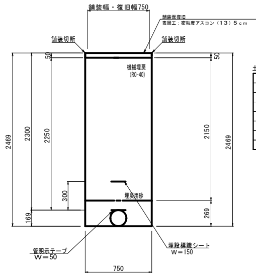
土工-1 (土被りH=2300) (DCPφ150) 矢板有り
