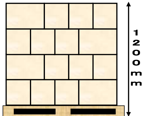
側面図
