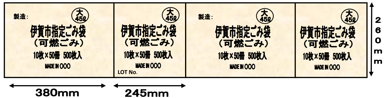
ダンボール箱仕様図
