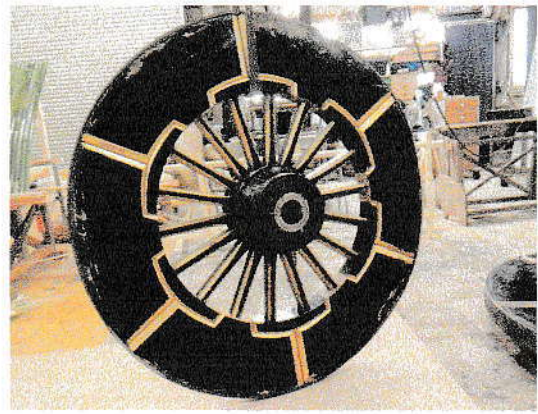
前右車輪（修理後）
