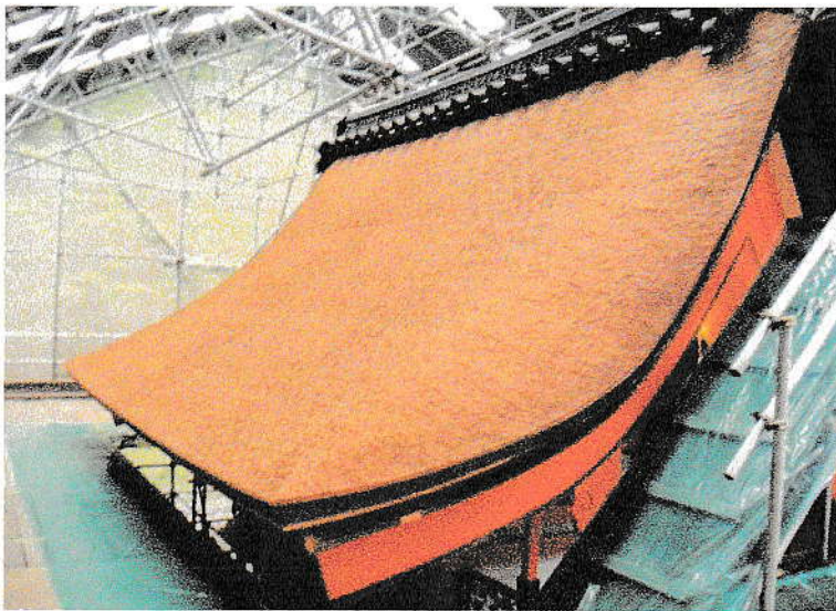
重文猪田神社本殿 檜皮屋根 葺替後
