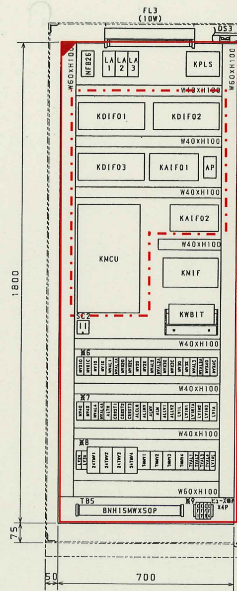
正面中板部品配置図
