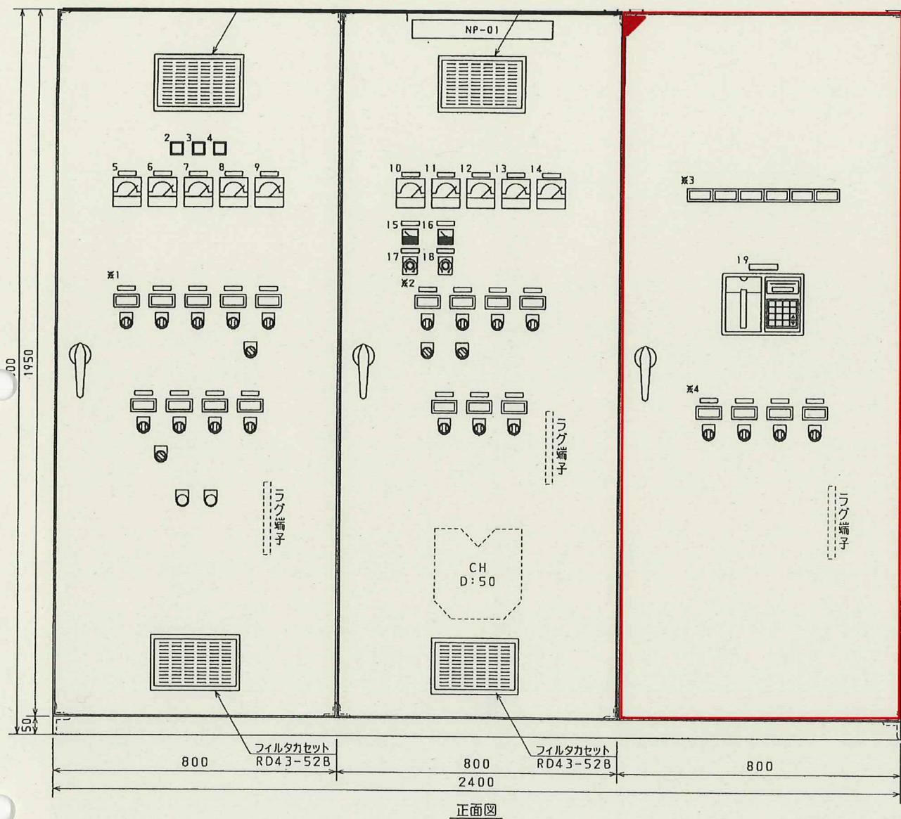
動力制御盤・計装盤
