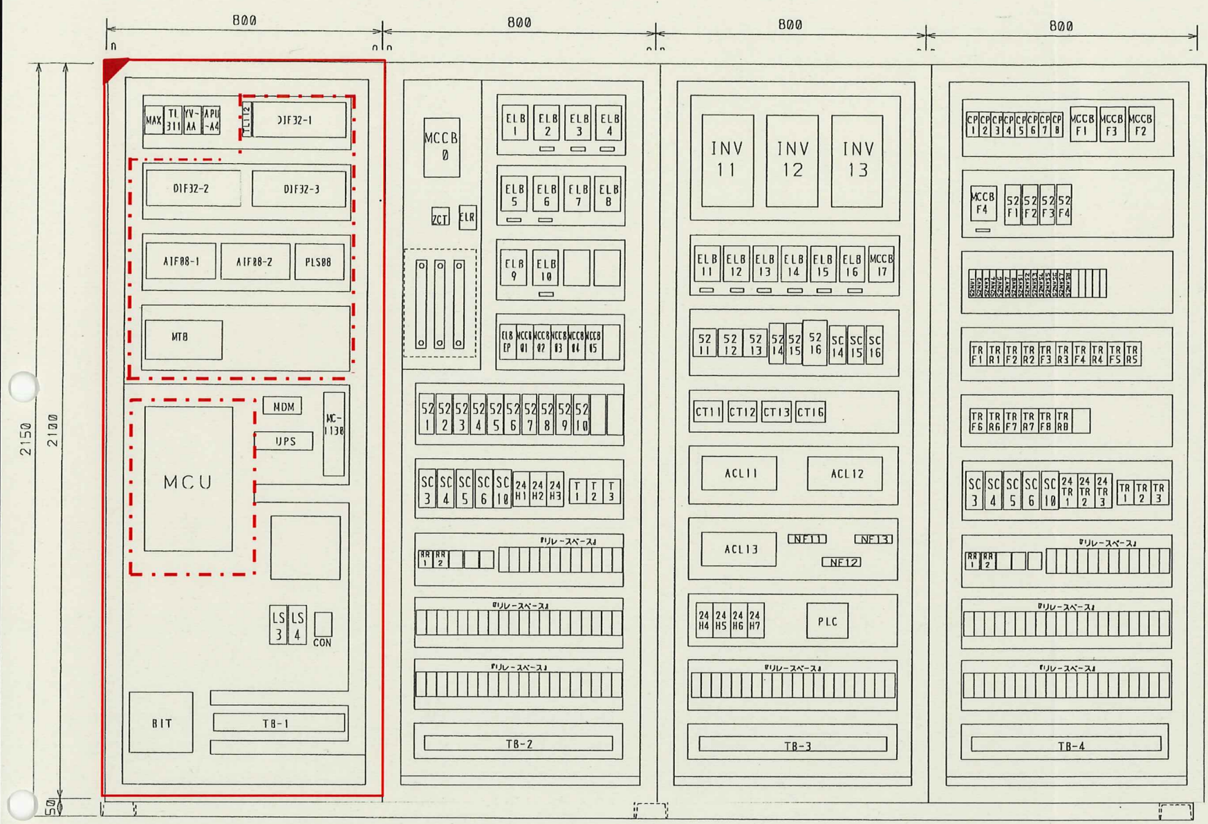
計装盤
