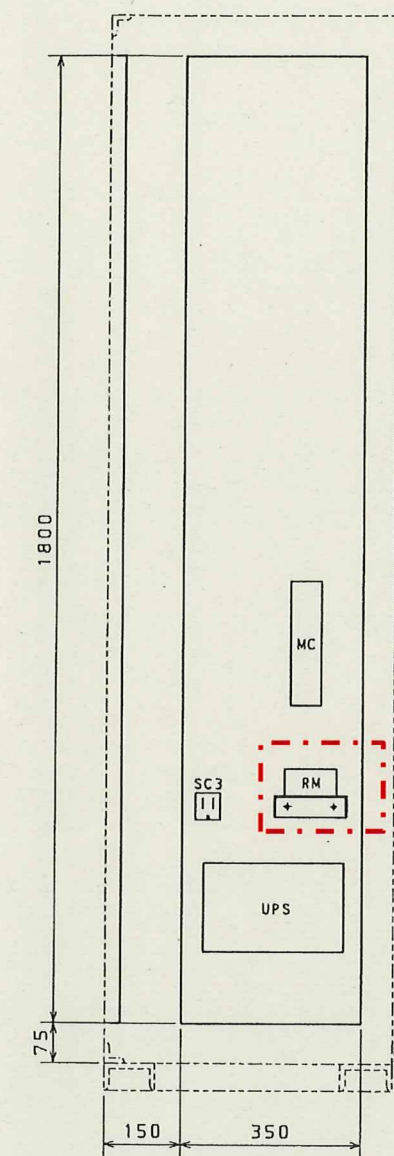
右側面中板部品配置図
