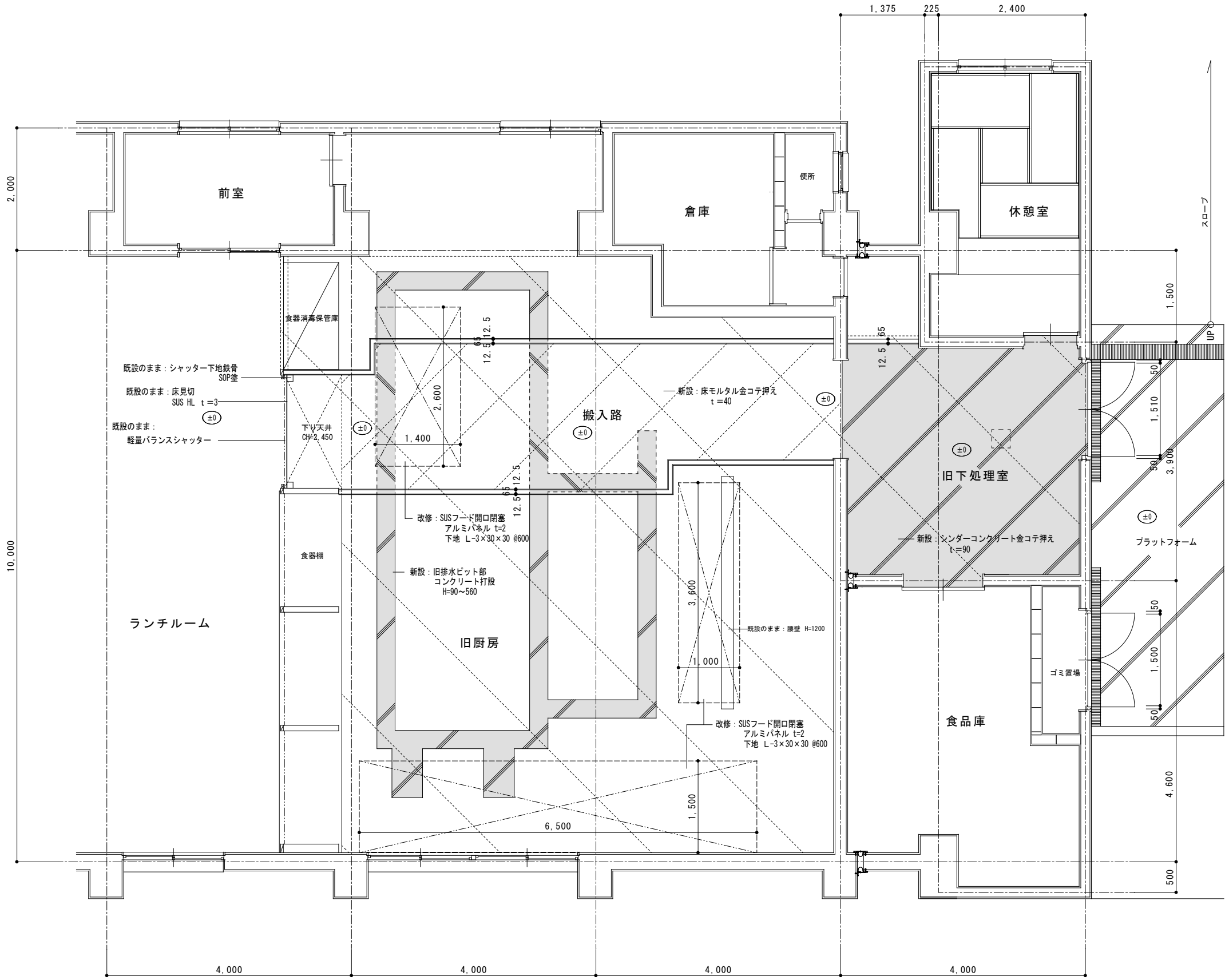
改修後 配膳室 平面図 S=1 : 50
