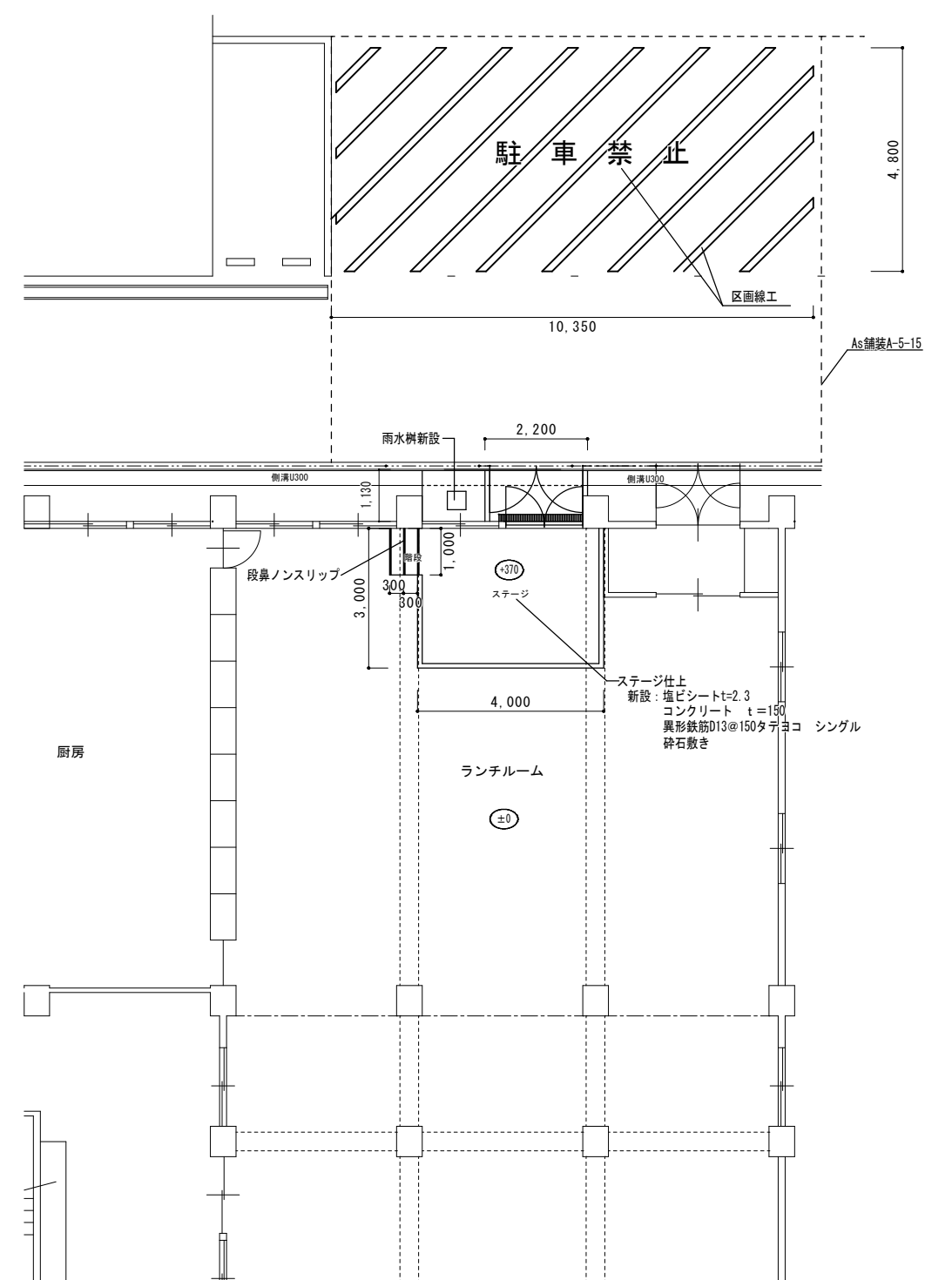
改修後 ランチルーム 平面図 S=1 : 100
