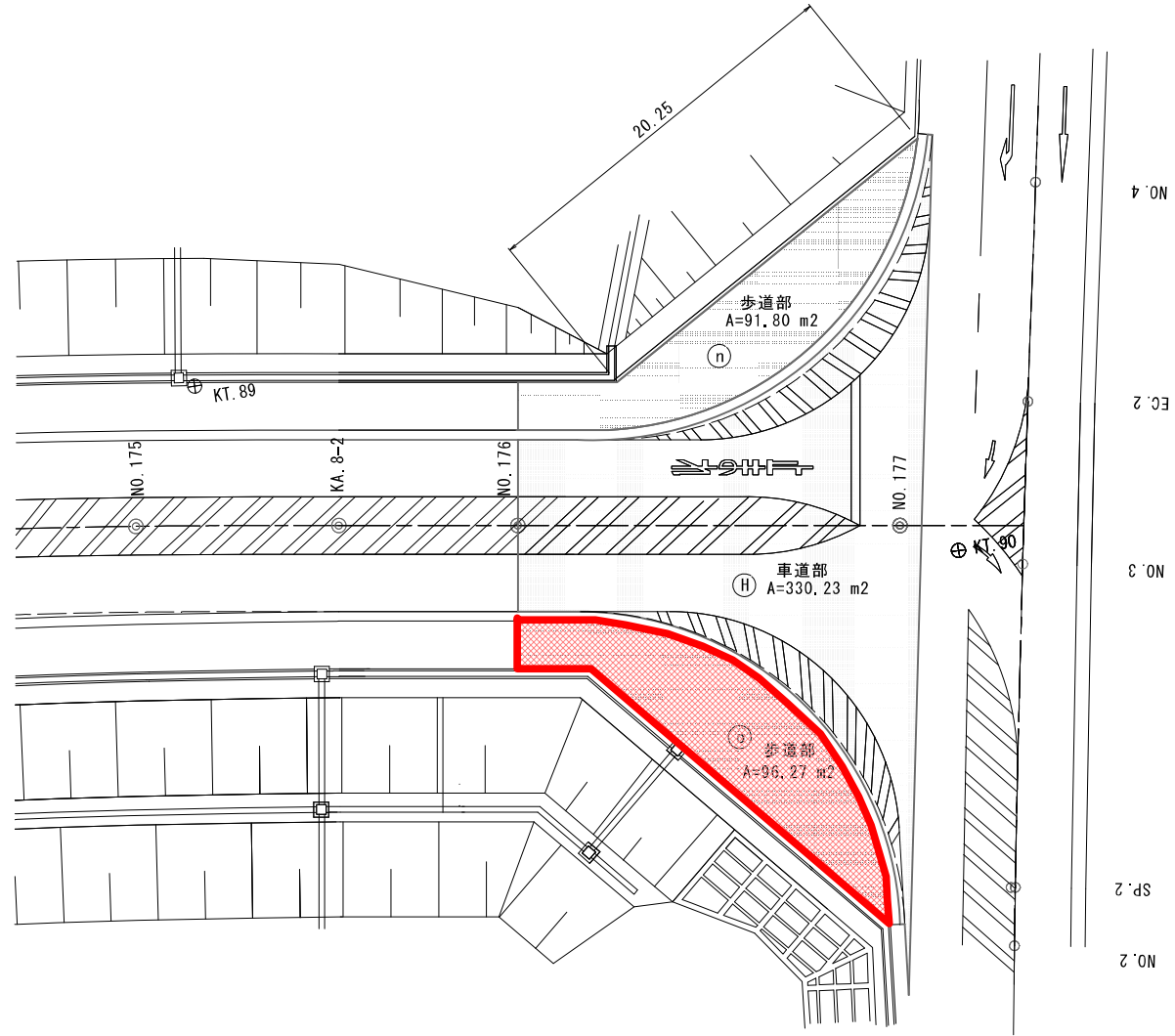
舗装根拠図
