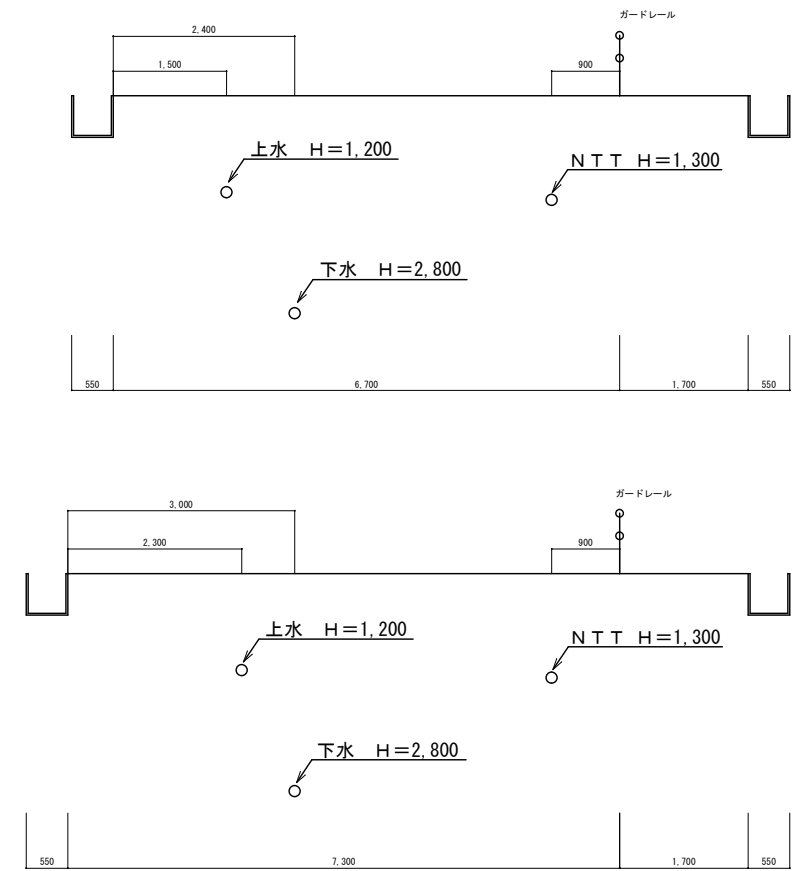
横断面図
