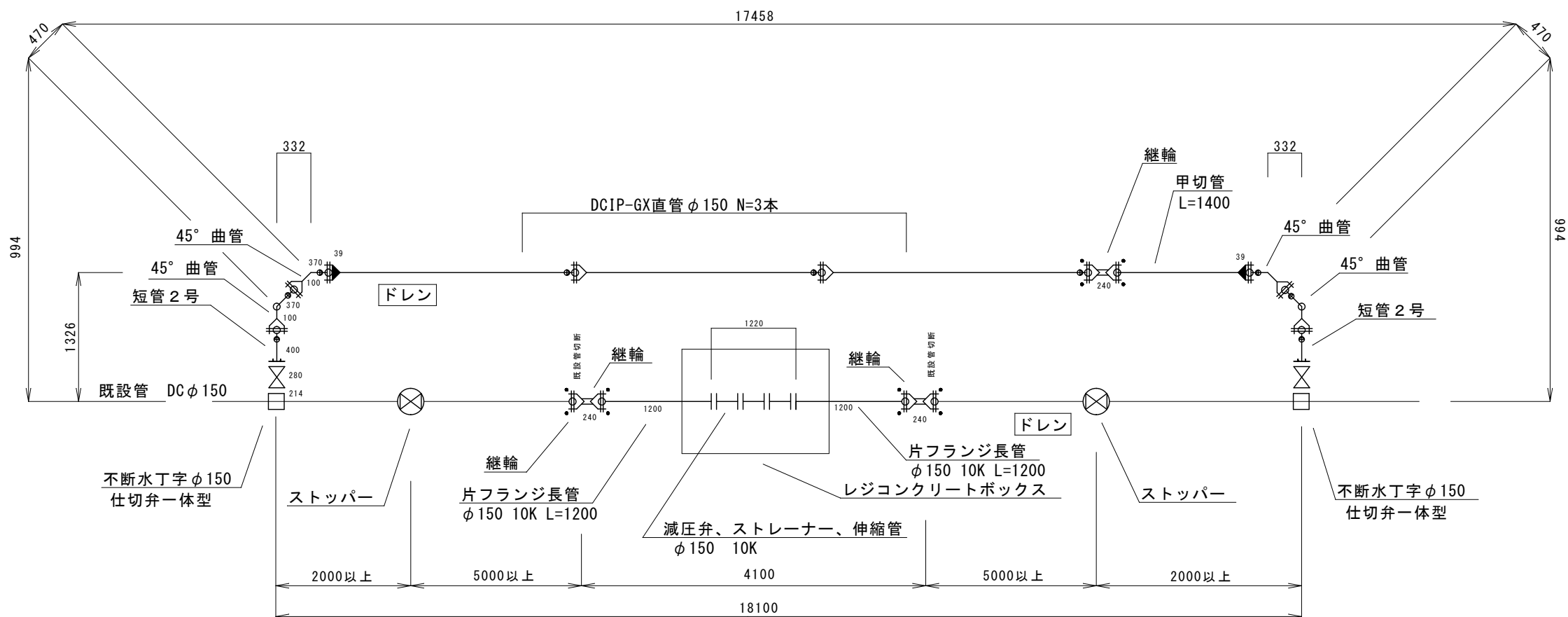
配管詳細図
