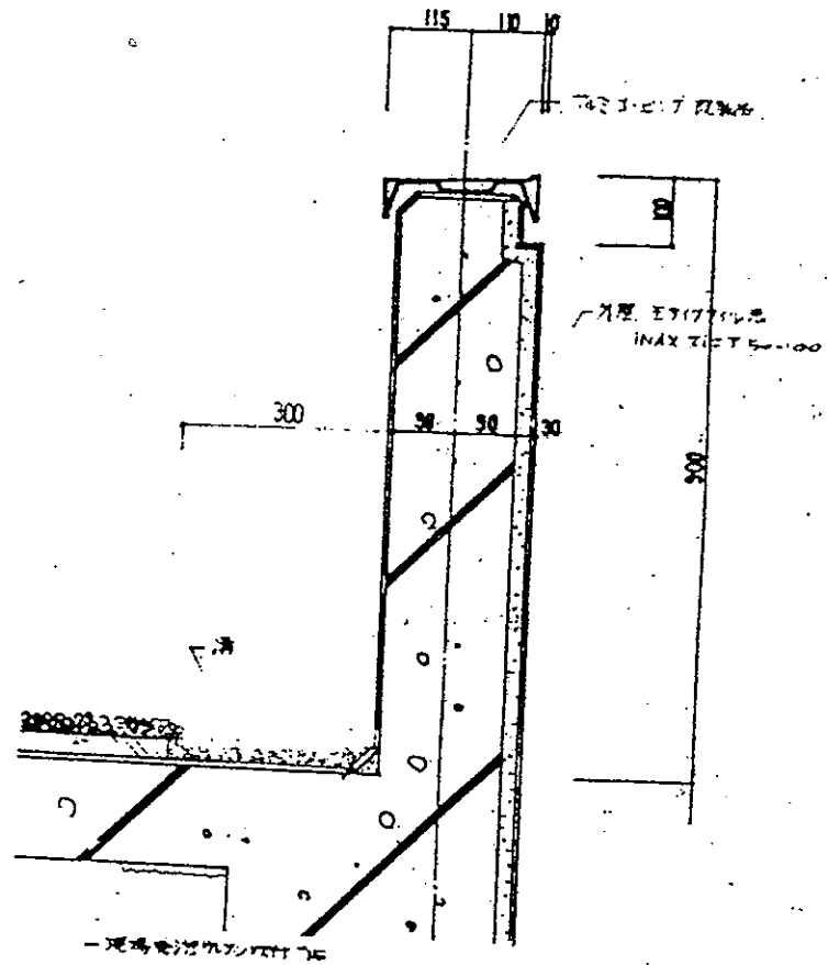
D-7 大正丸 新台 高層部 外壁部
