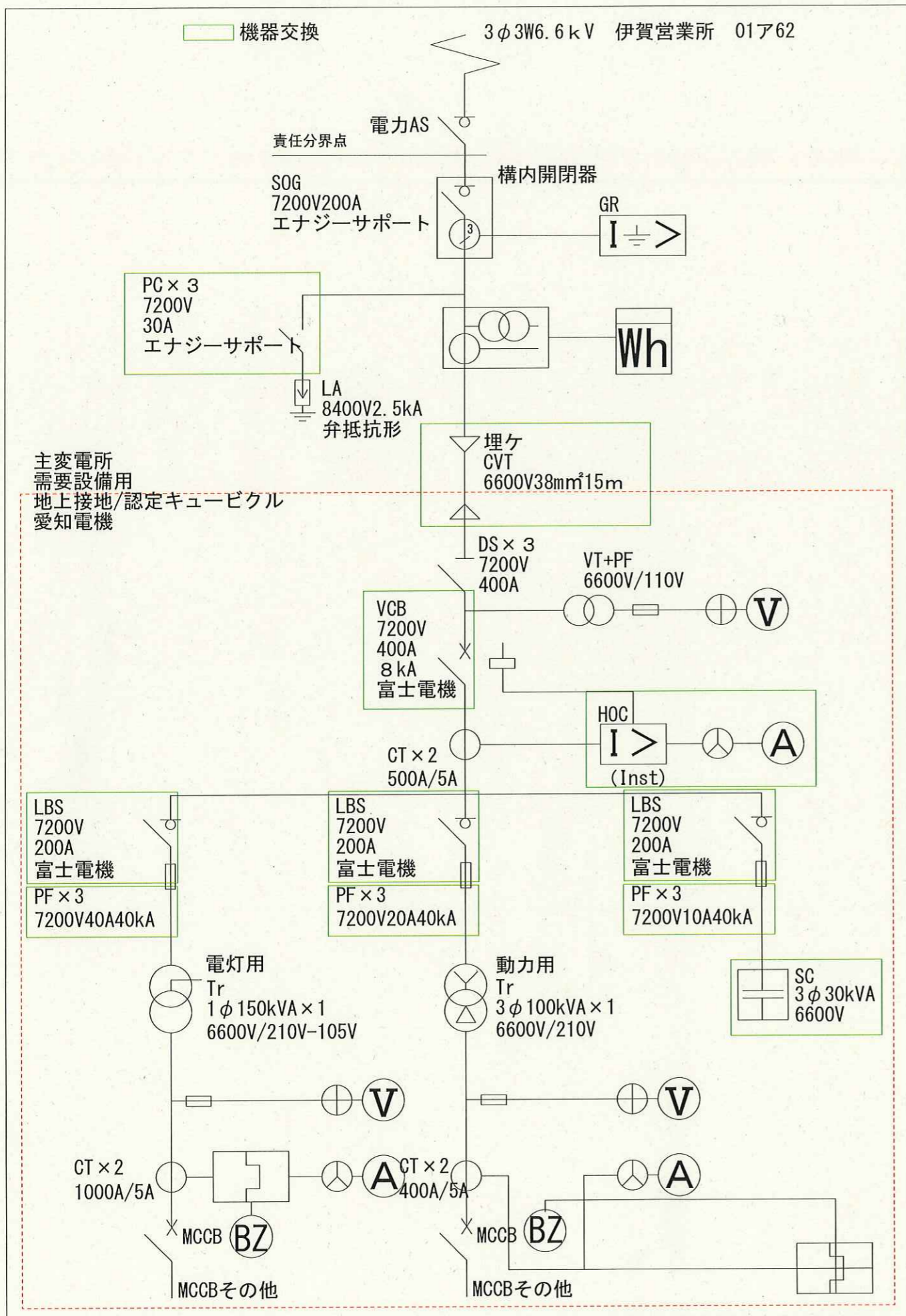
既設単線結線図 (上野西小学校)
