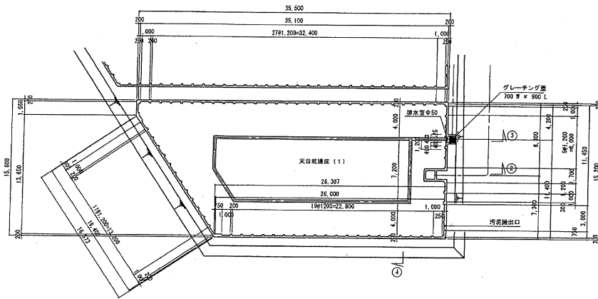
1 - 1 断面図 S=1:200
