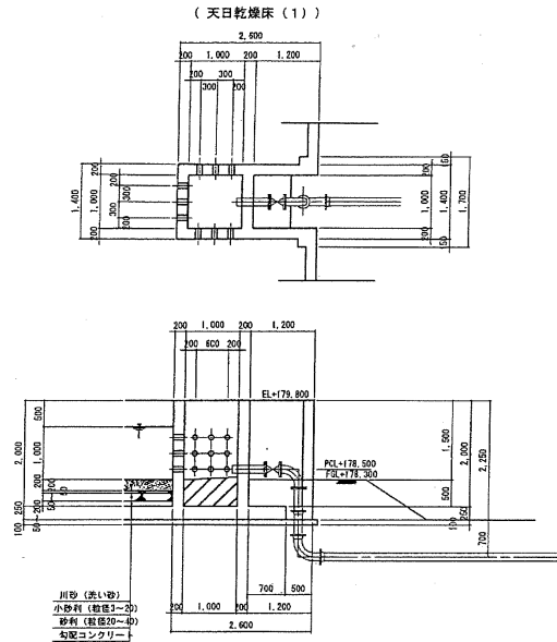
2 - 2 断面図 S=1:50
