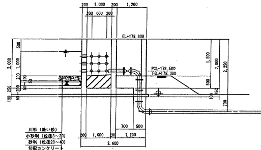
(天日乾燥床 (3))
