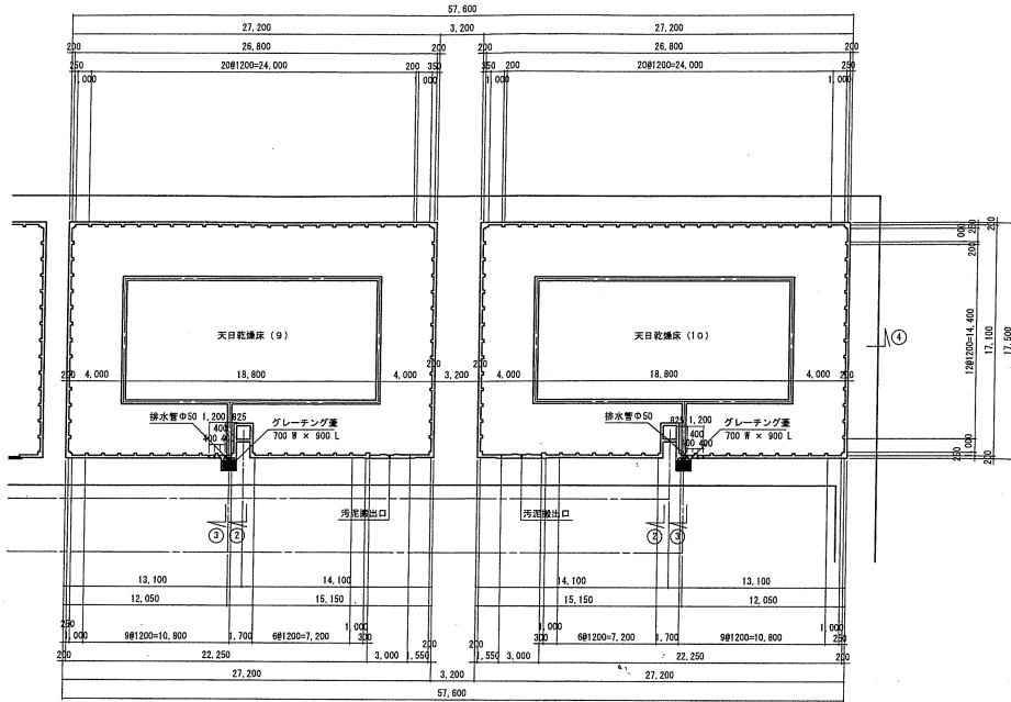
排水管展開図 S=1:50
