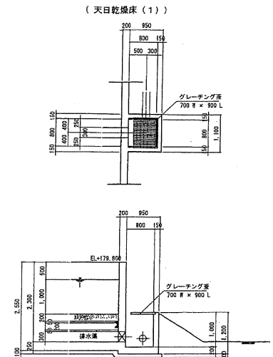
3 - 3 断面図 S=1:50
