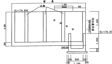
展開図
