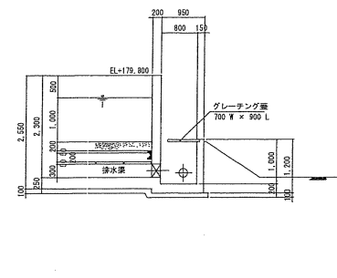
汚泥搬出口部断面図 S=1:50
