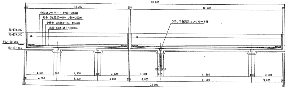
4-4 断面図 S=1:100
