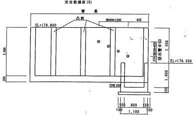
排水管展開図 S=1:50
