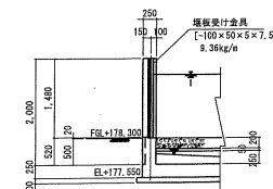
汚泥搬出口部断面図 S=1:50
