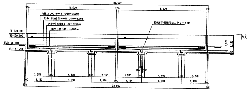
4-4 断面図 S=1:100
