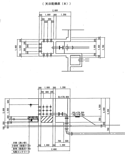
2 - 2 断面図 S=1:50
