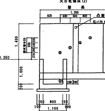
排水管展開図 S=1:50
