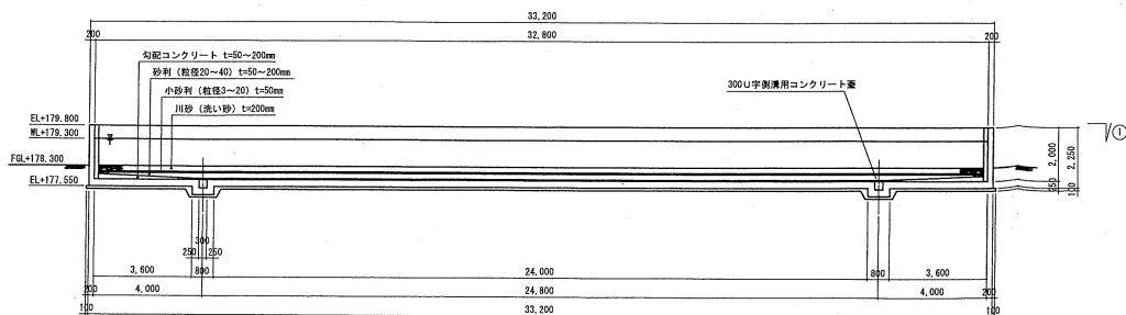
4 - 4 断面図 S=1:100
