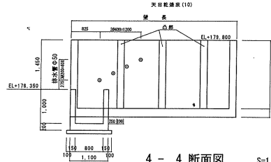
4 - 4 断面図 S=1:100
