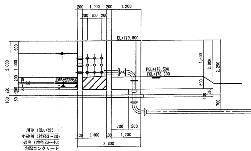
排水管展開図
