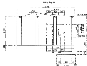
排水管展開図 S=1:50
