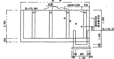
排水管展開図 S=1:50
