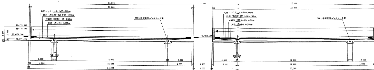
4 - 4 断面図 S=1:100
