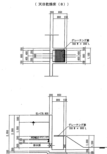
3 - 3 断面図 S=1:50
