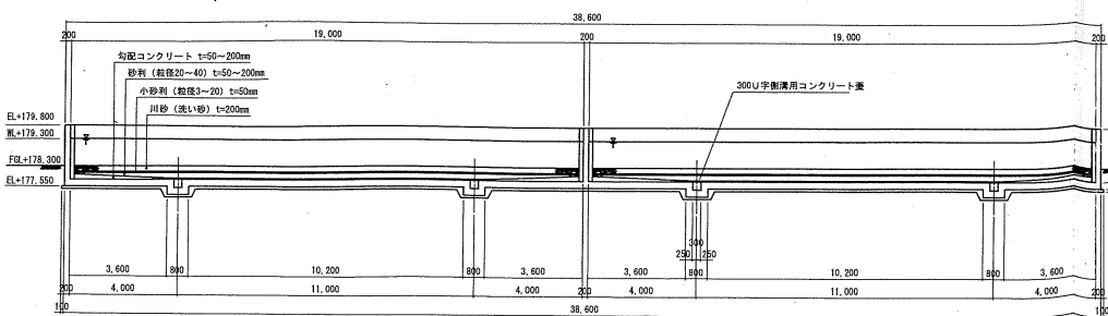
4 - 4 断面図 S=1:100
