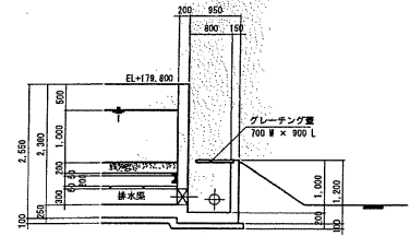
汚泥搬出口部断面図 S=1:50
