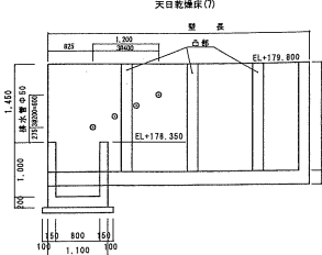
排水管展開図
