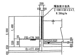
汚泥搬出口部断面図 S=1:50
