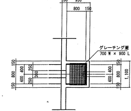
(天日乾燥床(10))
