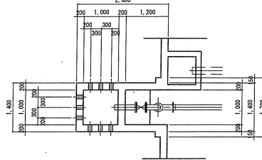
(天日乾燥床(10))
