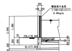
汚泥搬出口断面図 S=1:50
