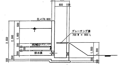
汚泥搬出口部断面図 S=1:50
