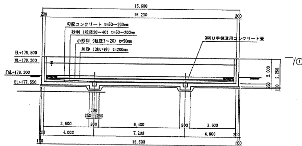
4 - 4 断面図 S=1:100
