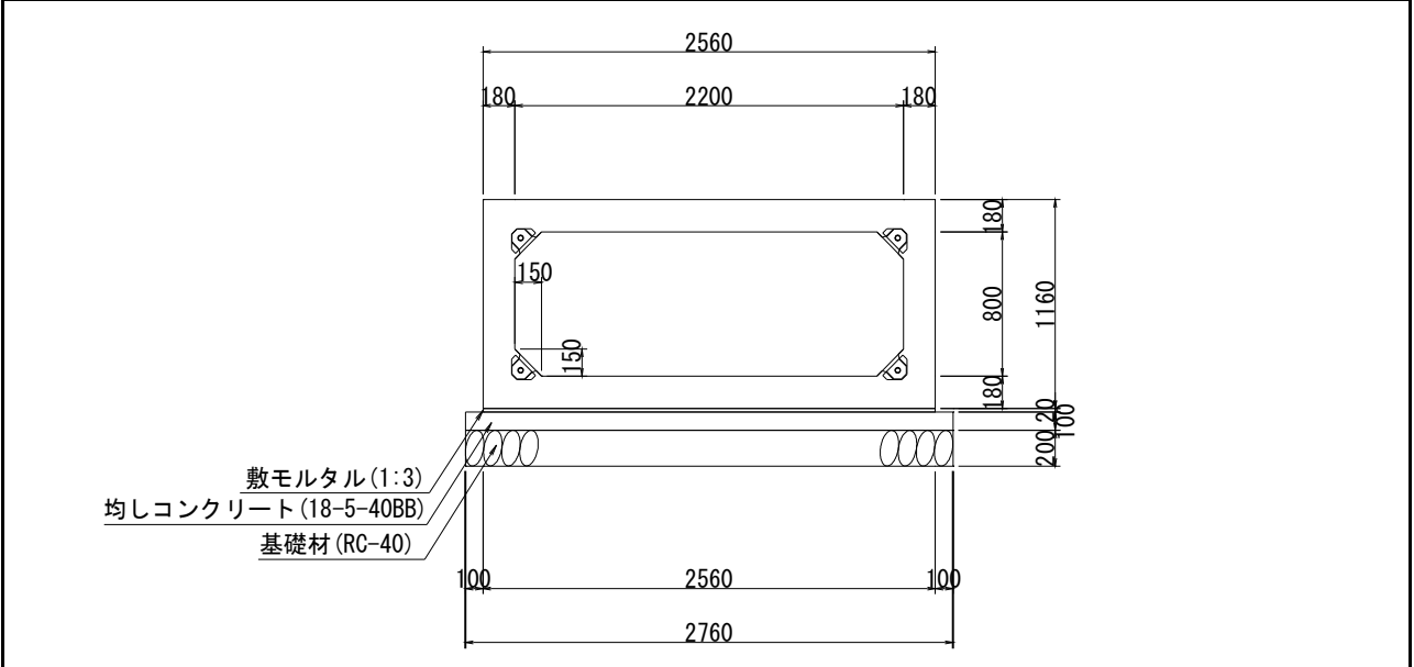
略 図
