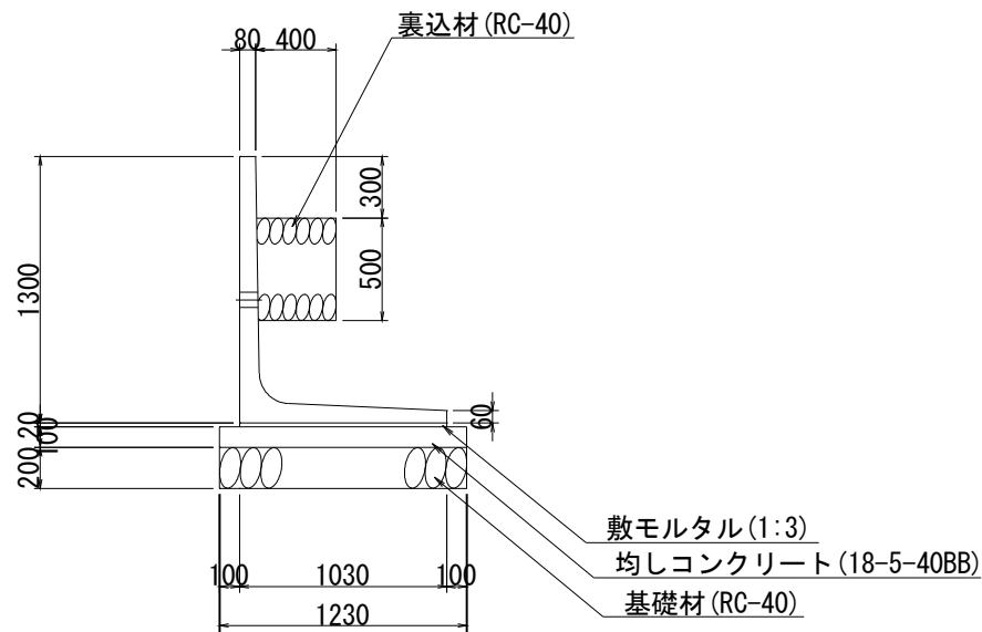
略 図
