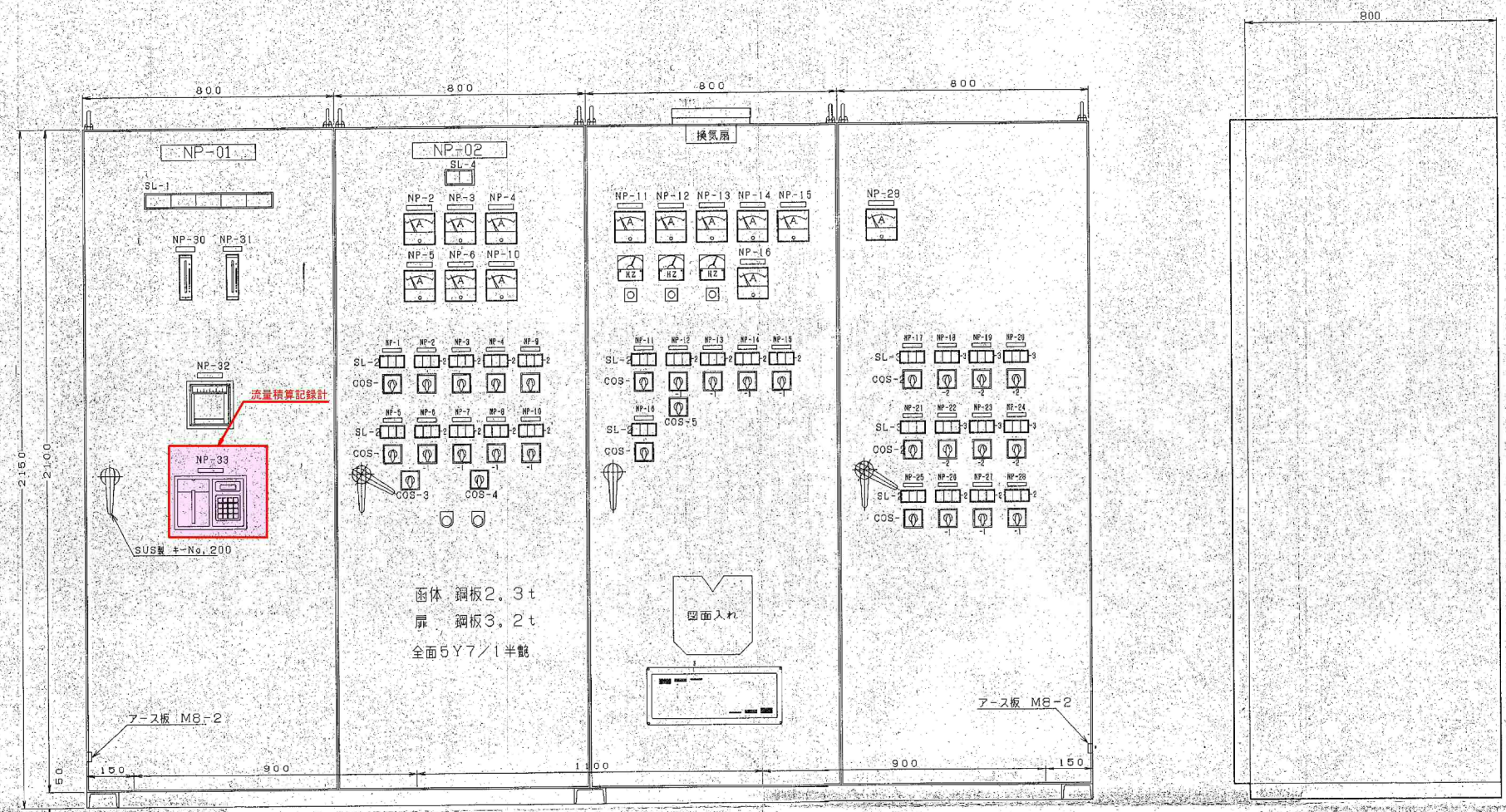
正面図 (S=1:10)
