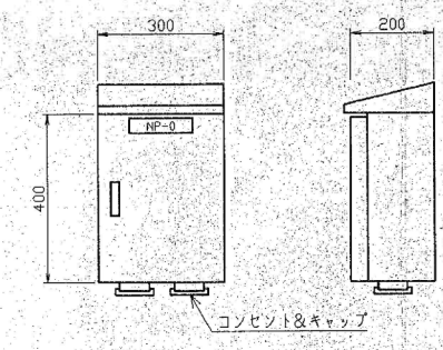
屋外壁掛型 可搬汚泥ポンプ用電源箱 (材質: SUS304) ※の外形寸法は参考とする。
