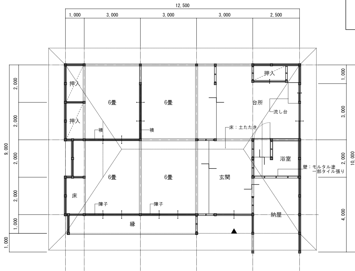
平面図 S=1: 100
