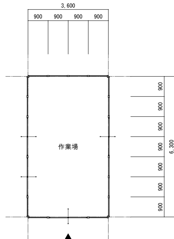
平面図 S=1: 100
