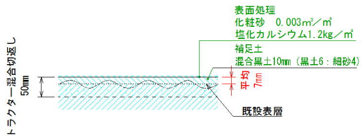
内野舗装断面図 1 : 10
