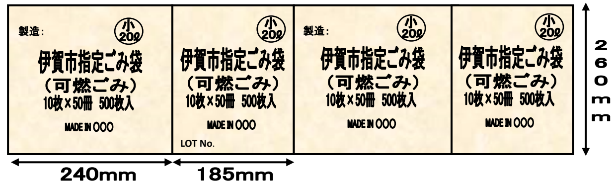
ダンボール箱仕様図
