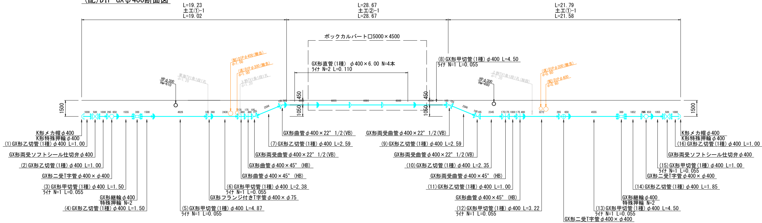
(配)DIP-GXφ400断面図
