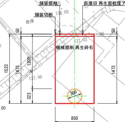
送水管φ300撤去断面図 土工⑥-3 S=1:25
