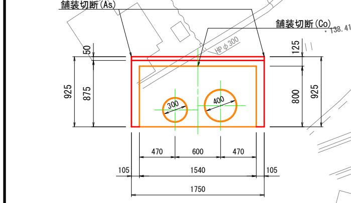
防護コンクリート撤去断面図 土工⑥-1 S=1:25
