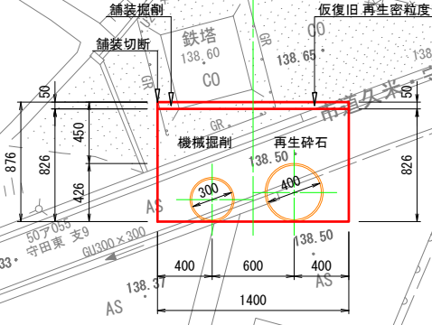
送水管φ300 配水管φ400同時撤去断面図 土工⑥-2 S=1:25
