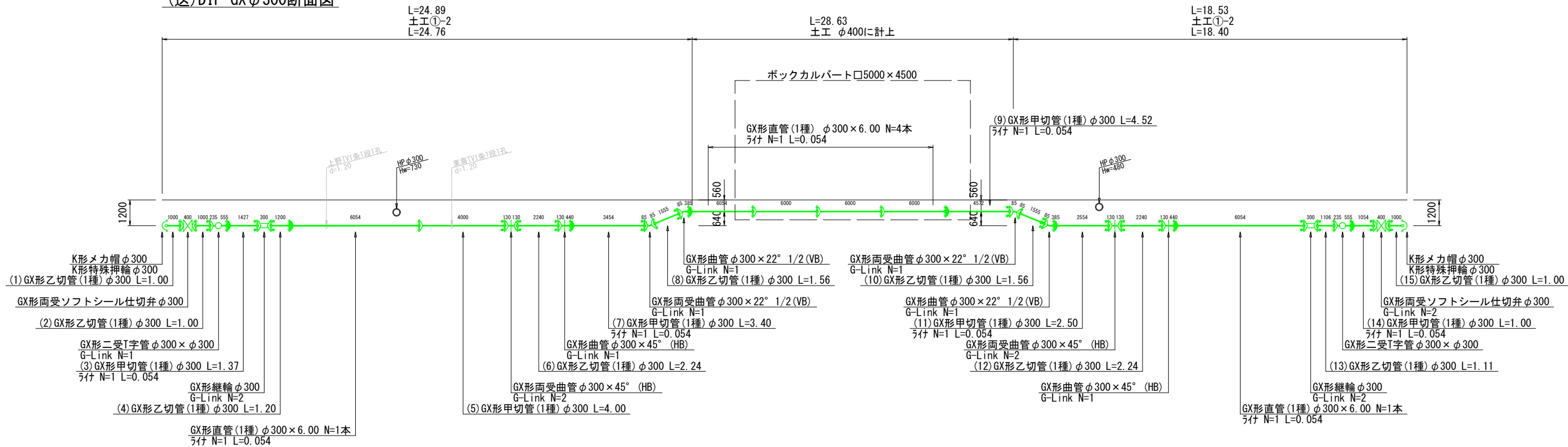
(送)DIP-GXφ300断面図
