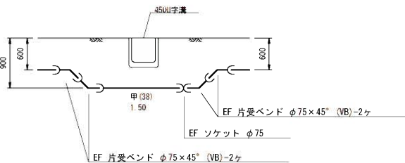
F-F断面図
