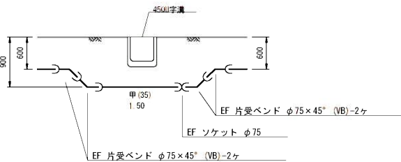
E-E断面図
