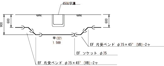
D-D断面図
