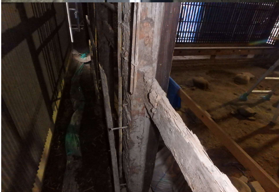
木部状況 北側柱 腐朽状況
