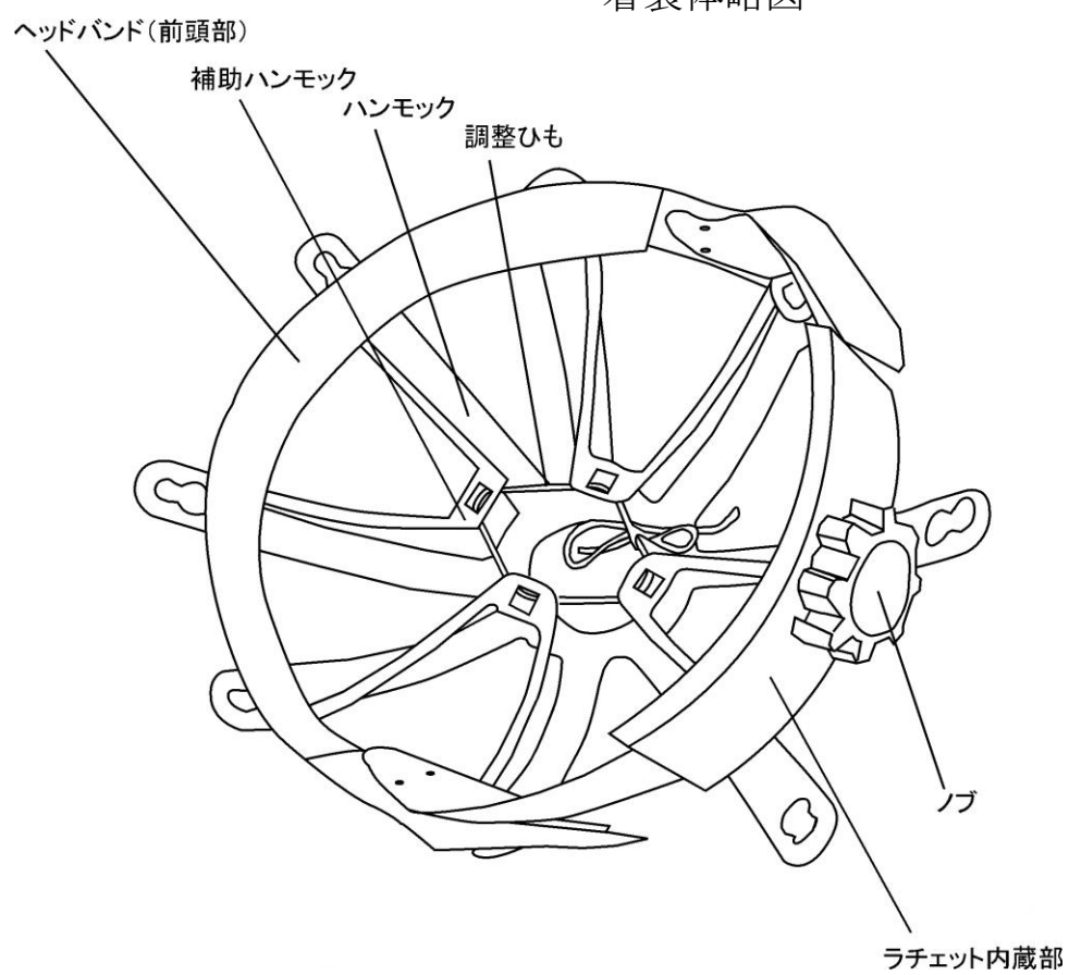
着装体略図
