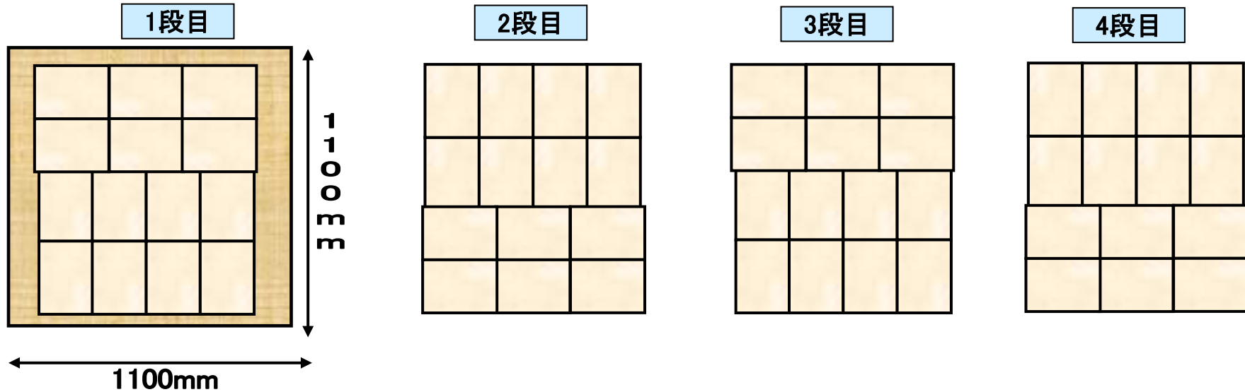
パレット積載図(1パレット56箱)
