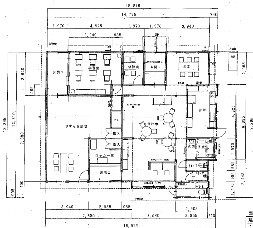
1階平面図
