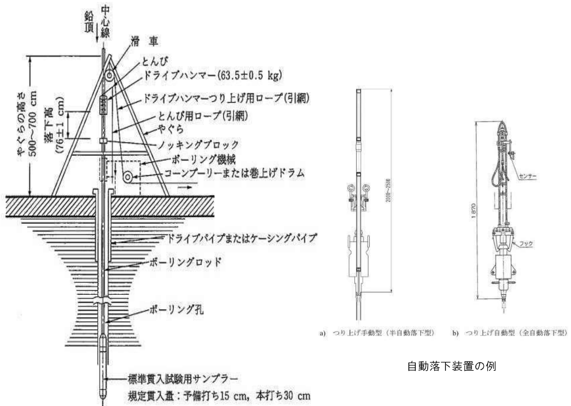
図2-2 標準貫入試験用サンプラー
