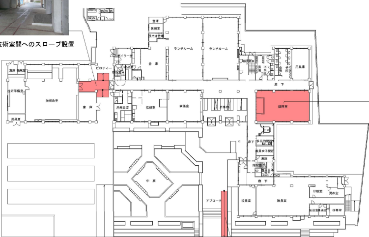
1階平面図
