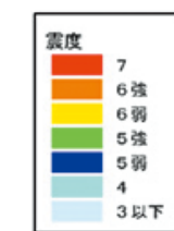
南海トラフ地震の震度予想図 (出典：気象庁ホームページ)
