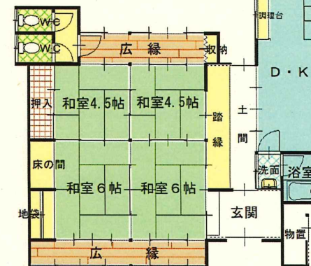
1 階 平 面 図
