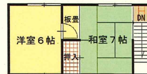
2 階 平 面 図
