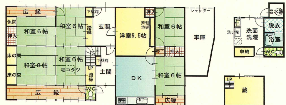
1階平面図
