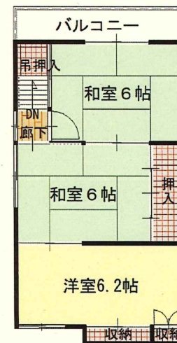
2階平面図
