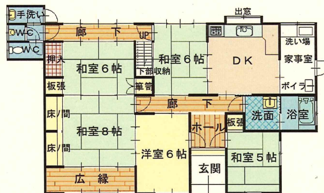
1階平面図
