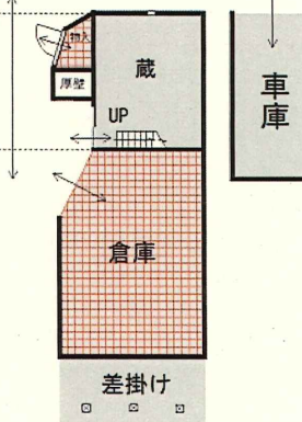
1F平面図
