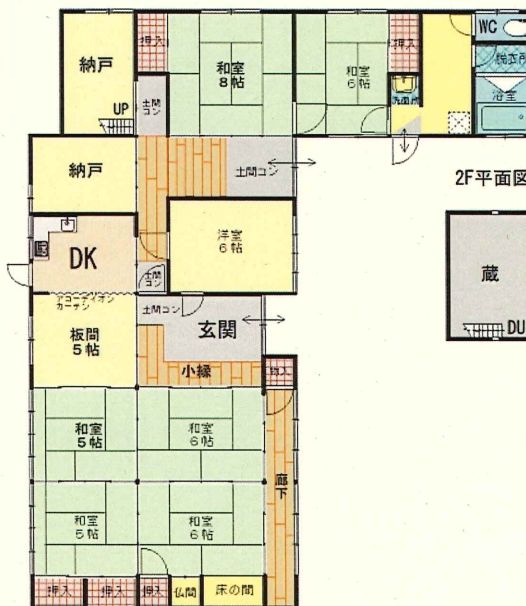
1F平面図
