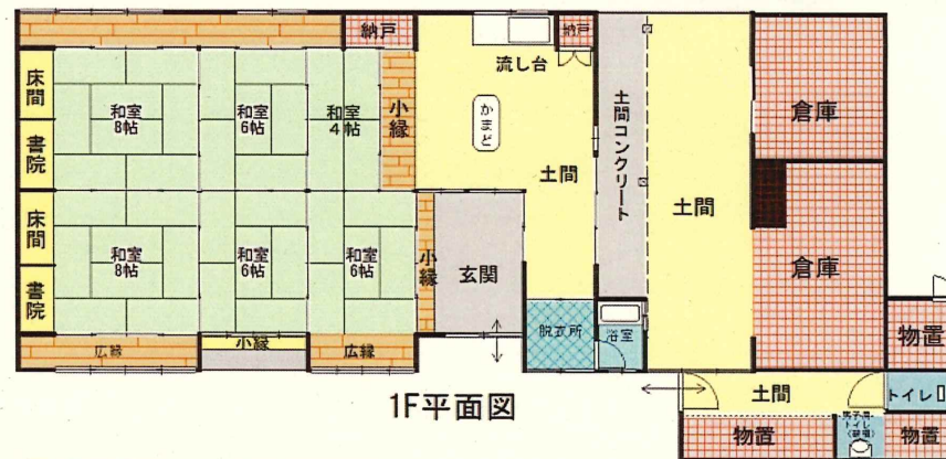
蔵 1F平面図
