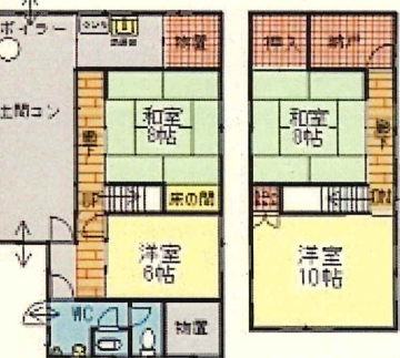
2F平面図
