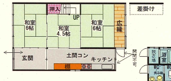
1F平面図
